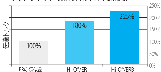
クランプナットの締め付けトルク比較表
