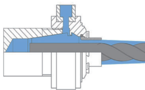
KS/ER クーラントフラッシュディスク装着例
