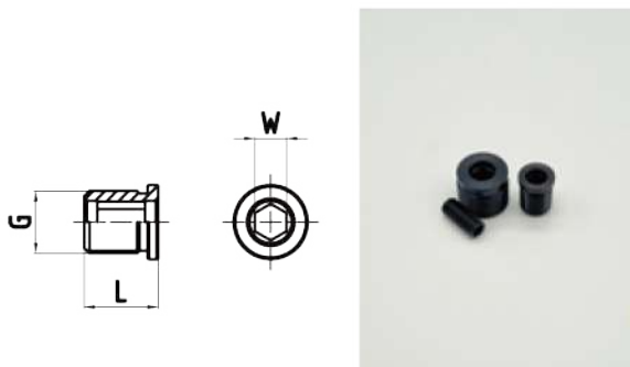
＝寸法 (mm)
