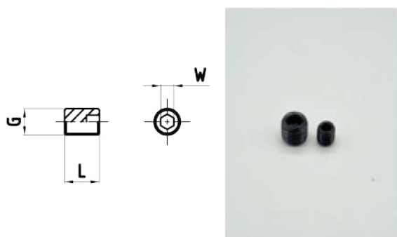
＝寸法 (mm)
