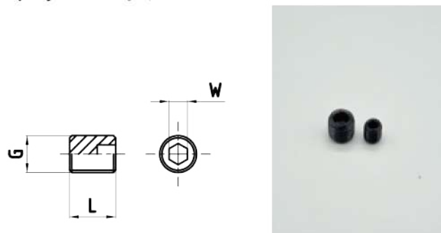
＝寸法 (mm)
