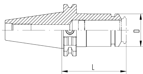
SK/PG ( A+AD型 )
