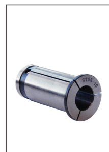
5-0949 1個 コレット C25-16
