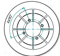
全てのコレットサイズに φ1.5mm x 4つのクーラント供給口
