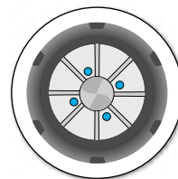
従来のERコレットにクーラント供給口を追加して潤滑性を向上
